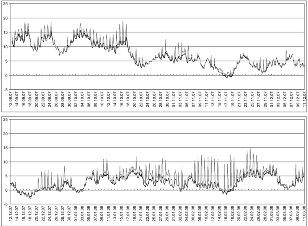
Abb. 4a: Temperaturverlauf im Untersuchungsgebiet 1 (Chilchberg) je 30 Meter nördlich (schwarz) oder südlich (grau) der Krette. Temperaturmessung alle drei Stunden. Winterhalbjahr vom 12.9.2007 bis 11.3.2008.
