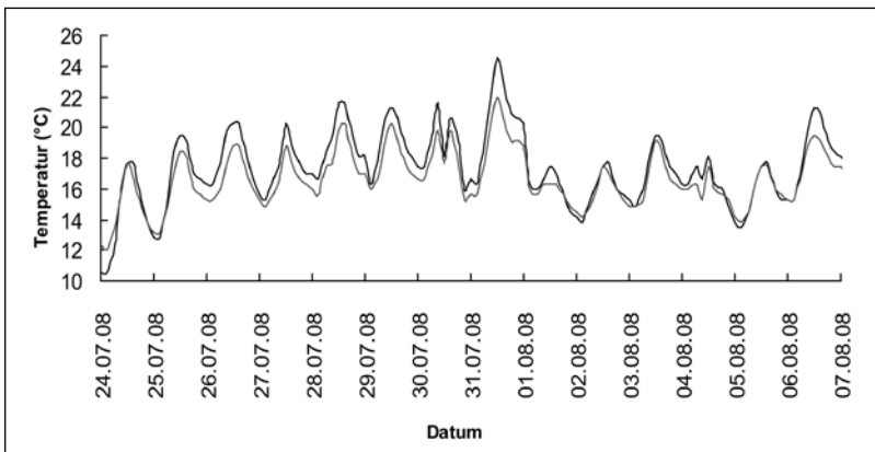
Abb. 6: Temperaturverlauf im Sommer in der obersten Streuschicht im Untersuchungsgebiet 2 (Riedberg). Messungen jeweils 5 Meter von der Krete im süd- (grau) oder nordgerichteten Hang (schwarz).
