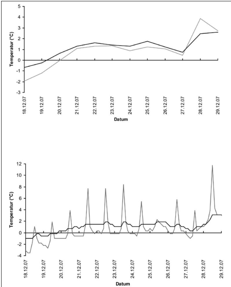
Abb. 5: Temperaturverlauf (18. 12. 07–29. 12. 07) in der obersten Streuschicht im Untersuchungsgebiet 1 (Chilchberg). Messungen jeweils 5 Meter von der Krete im süd- (grau) oder nordgerichteten Hang (schwarz). Unten: effektive Messwerte im drei-Stunden-Intervall. Oben: Tagesmittelwerte.
